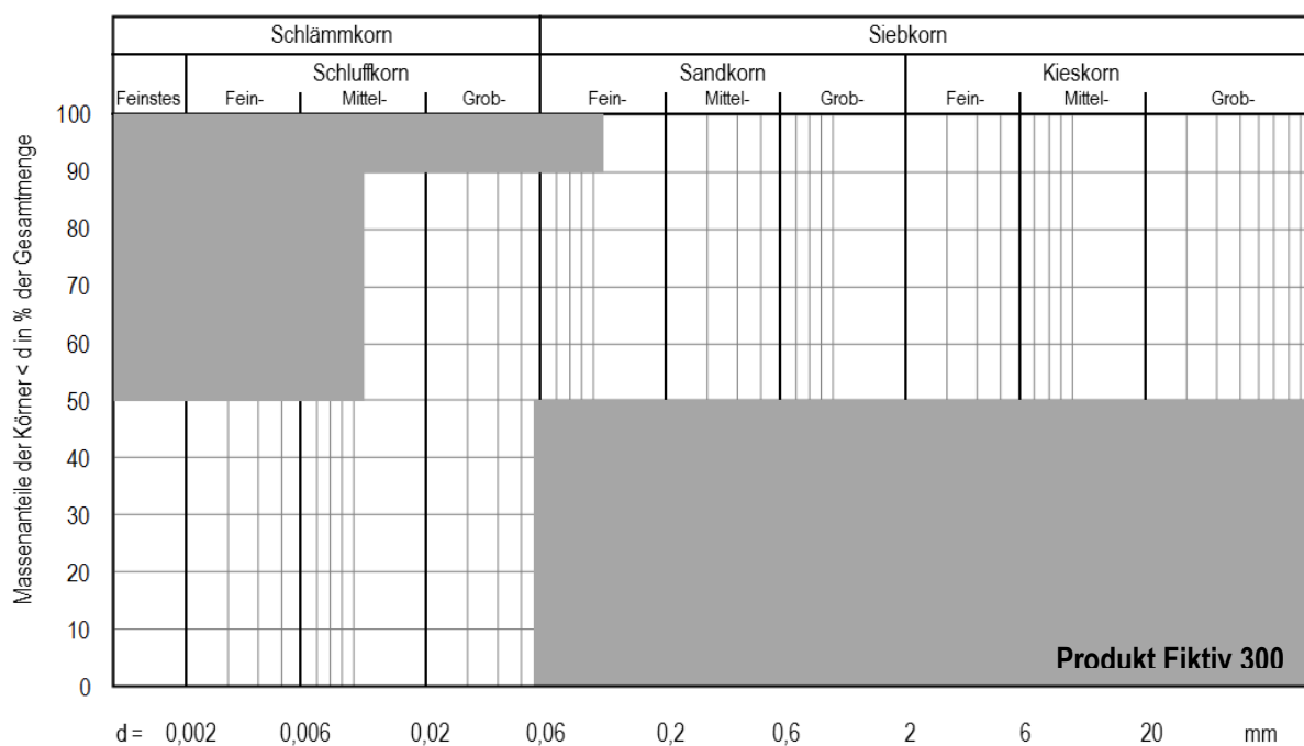
Zulässige Kornverteilungen Bild 1
