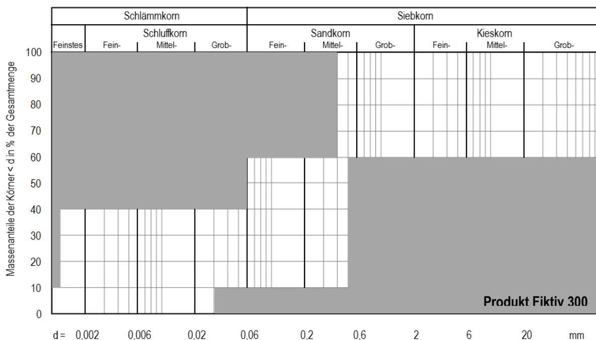
Zulässige Kornverteilungen Bild 9
