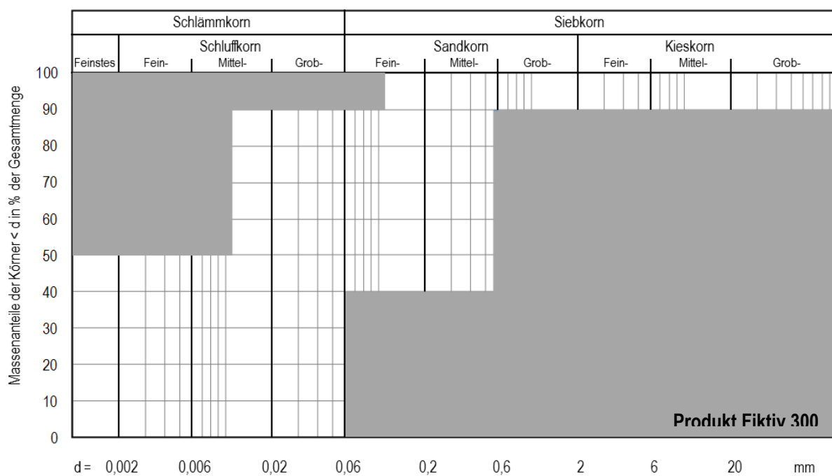
Zulässige Kornverteilungen Bild 2
